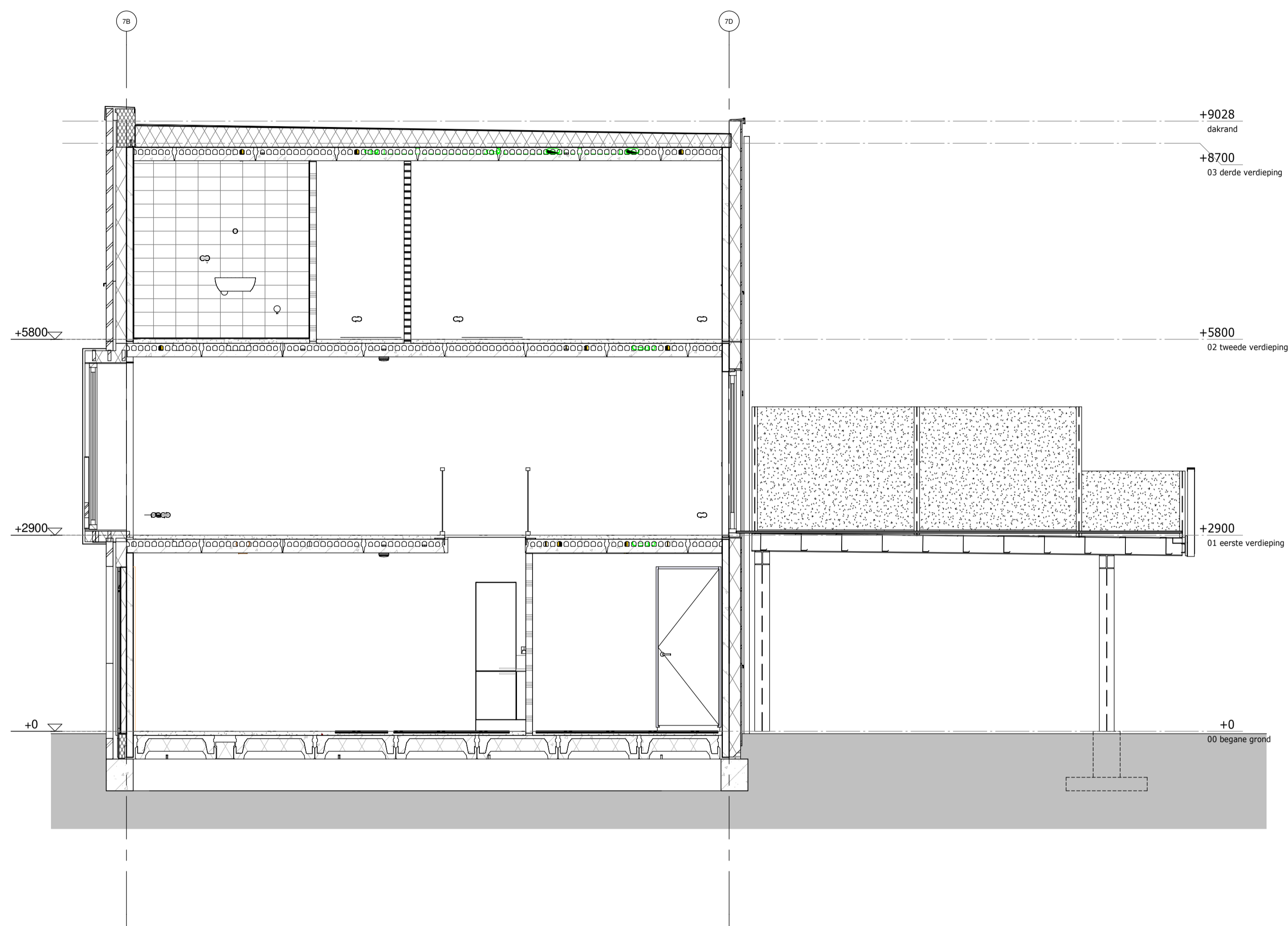
doorsnede 09c/c1
