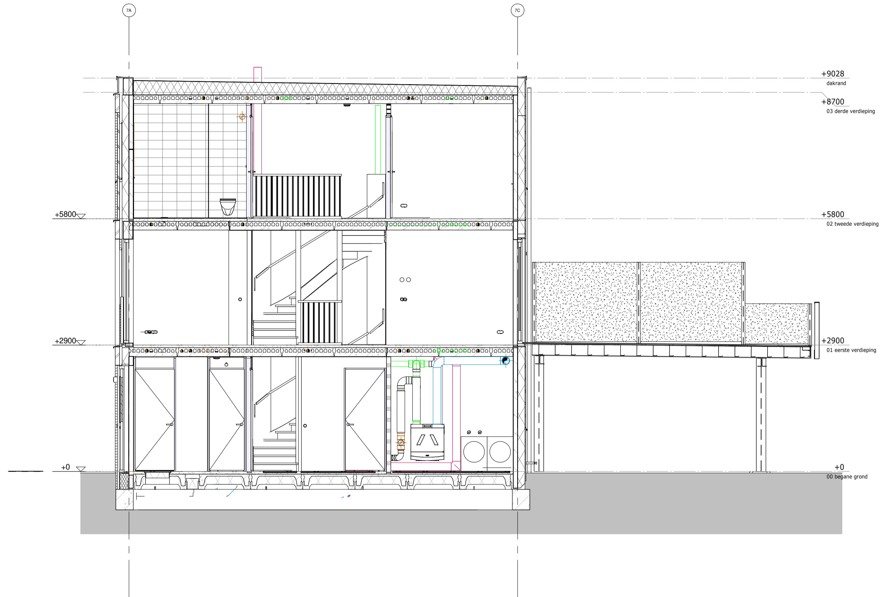
doorsnede 09d/c2
